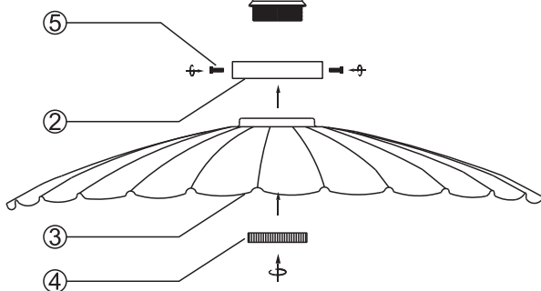
Рис.4 Сборка и установка светильника.
